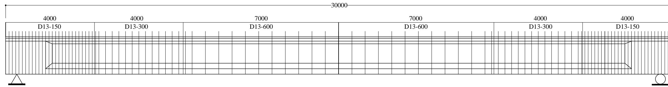
DETAIL TULANGAN GESER
