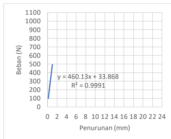
Grafik 9.5 Garis Bantu & R^2 KL-8mm-5
