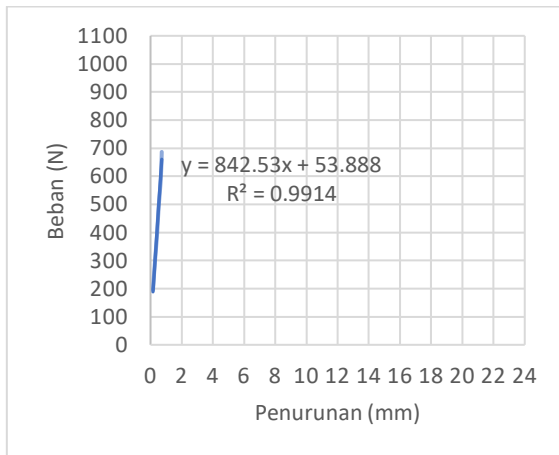
Grafik 9.1 Garis Bantu & R^2 KL-8mm-1
