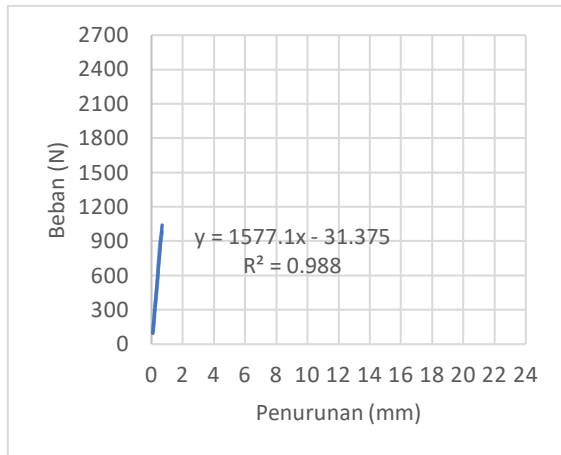
Grafik 9.6 Garis Bantu & R^2 KL-10mm-1
