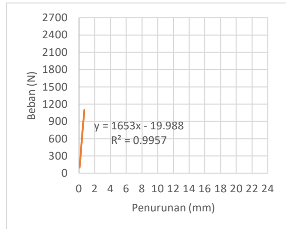
Grafik 9.7 Garis Bantu & R^2 KL-10mm-2
