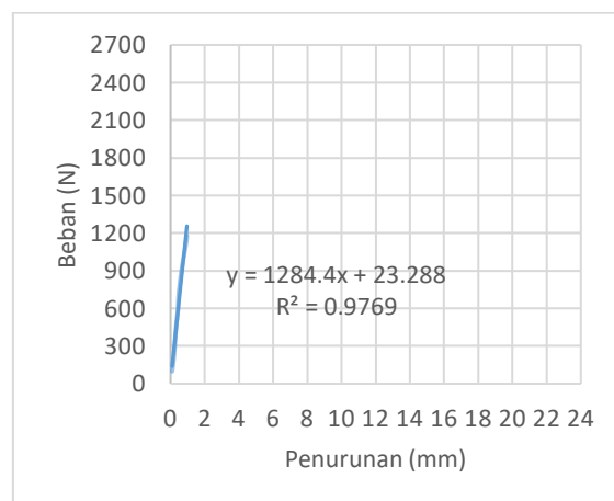
Grafik 9.10 Garis Bantu & R^2 KL-10mm-5
