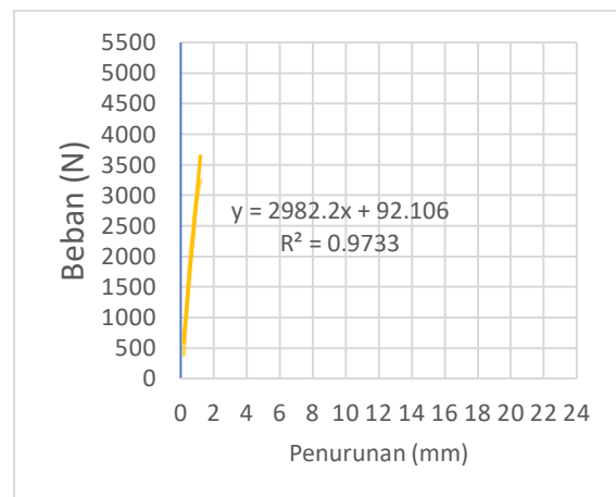
Grafik 9.13 Garis Bantu & R^2 KL-12mm-3 Grafik 9.14 Garis Bantu & R^2 KL-12mm-4
