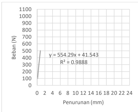
Grafik 9.3 Garis Bantu & R^2 KL-8mm-3
