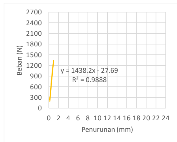
Grafik 9.9 Garis Bantu & R^2 KL-10mm-4
