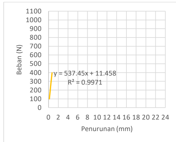
Grafik 9.2 Garis Bantu & R^2 KL-8mm-2
