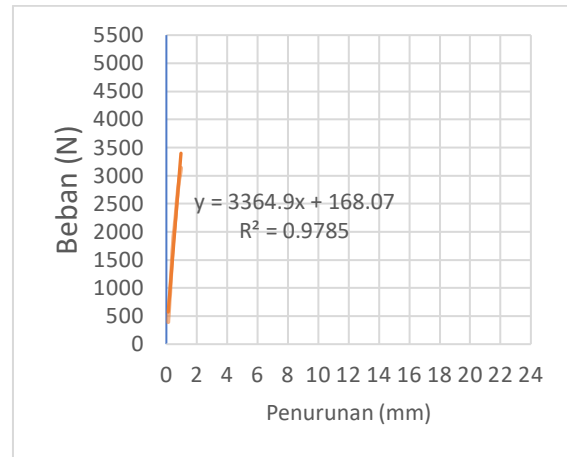
Grafik 9.11 Garis Bantu & R^2 KL-12mm-1 Grafik 9.12 Garis Bantu & R^2 KL-12mm-2
