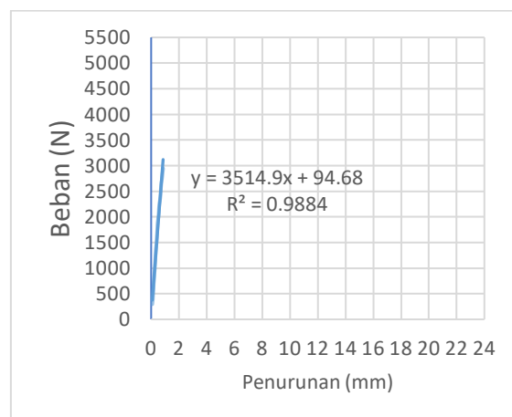
Grafik 9.15 Garis Bantu & R^2 KL-12mm-5
