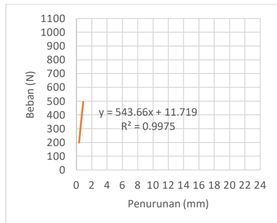
Grafik 9.4 Garis Bantu & R^2 KL-8mm-4
