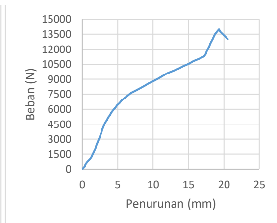
Grafik 8.12 Pengujian KS-10mm-5
