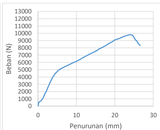
Grafik 8.6 Pengujian KS-8mm-5
