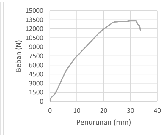
Grafik 8.10 Pengujian KS-10mm-3
