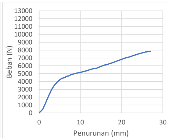
Grafik 8.2 Pengujian KS-8mm-1
