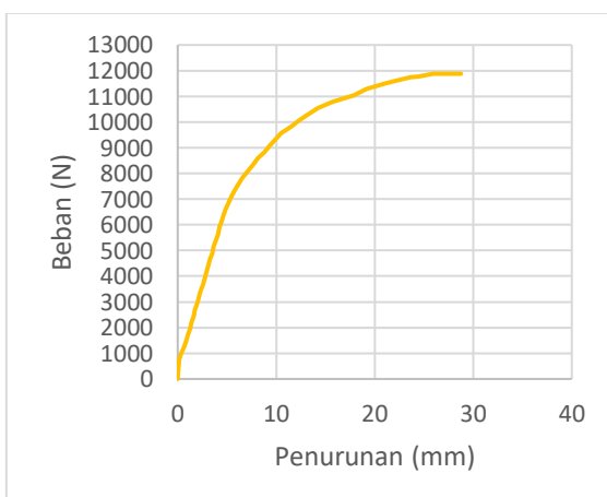
Grafik 8.17 Pengujiuan KS-12mm-4
