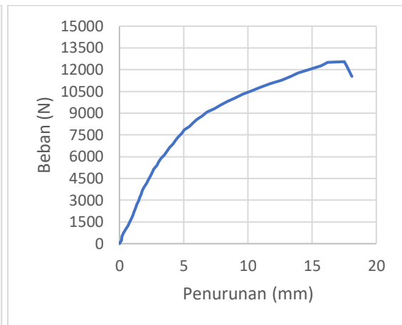
Grafik 8.8 Pengujian KS-10mm-1
