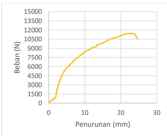
Grafik 8.11 Pengujian KS-10mm-4
