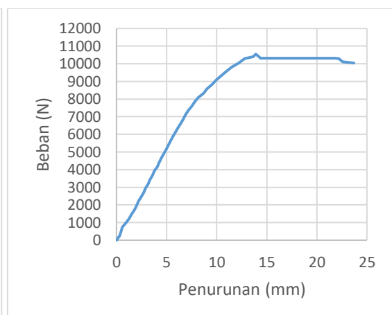
Grafik 8.18 Pengujiuan KS-12mm-5
