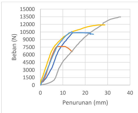
Grafik 8.13 Pengujiuan Kuat Sambung dengan Alat Sambung Baut 12mm
