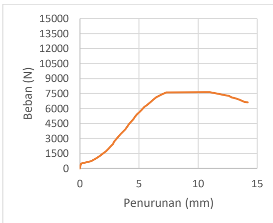
Grafik 8.15 Pengujiuan KS-12mm-2
