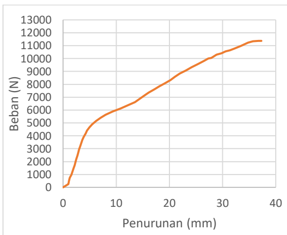
Grafik 8.3 Pengujian KS-8mm-2
