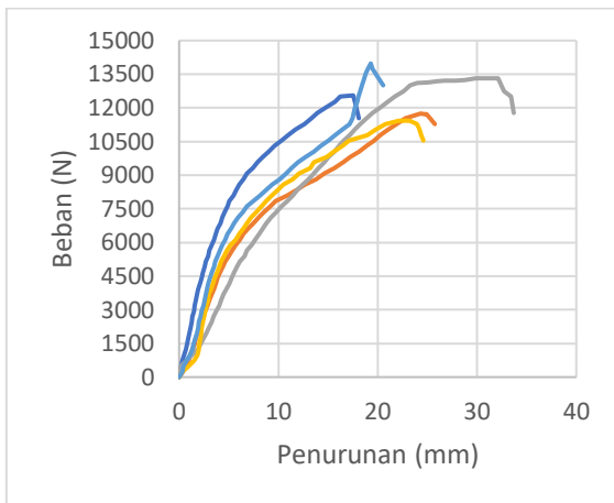
Grafik 8.7 Pengujian Kuat Sambungan dengan Alat Sambung Baut 10mm
