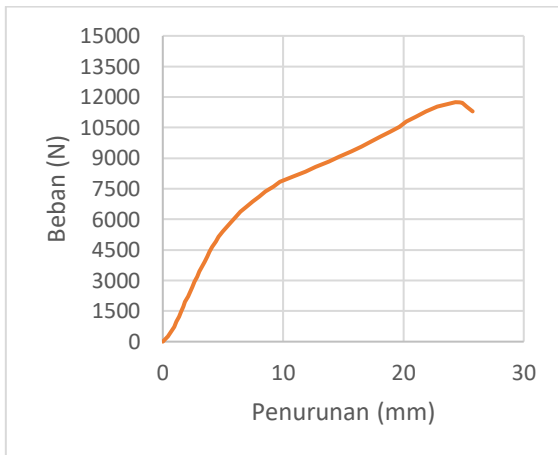
Grafik 8.9 Pengujian KS-10mm-2
