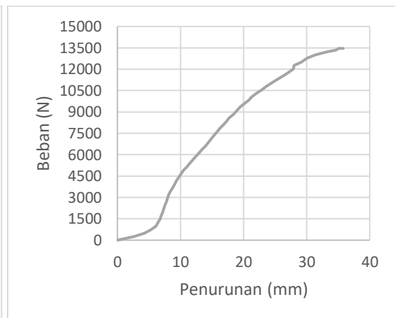
Grafik 8.16 Pengujiuan KS-12mm-3
