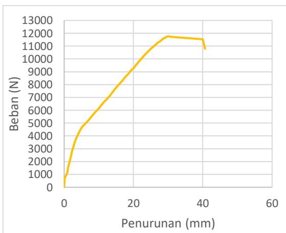
Grafik 8.5 Pengujian KS-8mm-4
