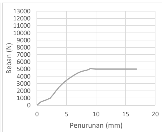
Grafik 8.4 Pengujian KS-8mm-3
