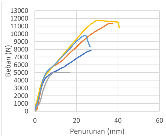
Grafik 8.1 Pengujian Kuat Sambungan dengan Alat Sambung Baut 8mm
