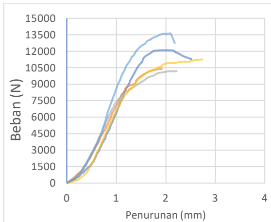
Grafik 7.1 Pengujian Kuat Tumpu dengan Baut Penekan 8mm
