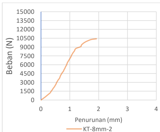
Grafik 7.3 Pengujian KT-8mm-2
