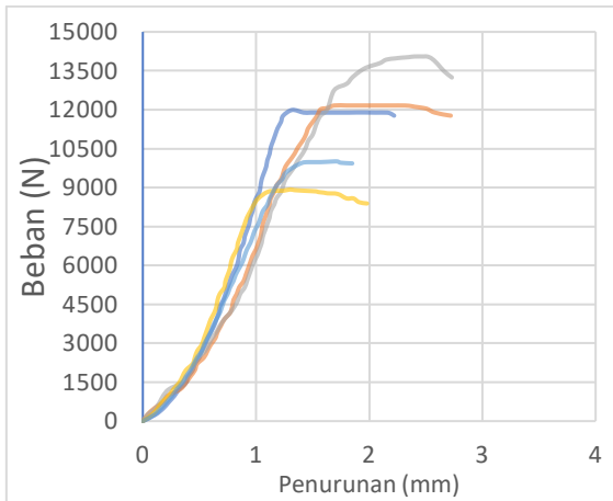
Grafik 7.7 Pengujian Kuat Tumpu dengan Baut Penekan 10mm
