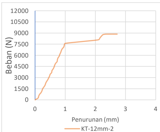
Grafik 7.15 Pengujiuan KT-12mm-2
