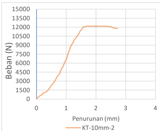
Grafik 7.9 Pengujian KT-10mm-2
