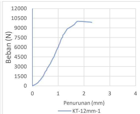
Grafik 7.14 Pengujiuan KT-12mm-1
