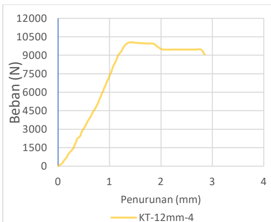
Grafik 7.17 Pengujiuan KT-12mm-4
