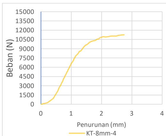
Grafik 7.5 Pengujian KT-8mm-4
