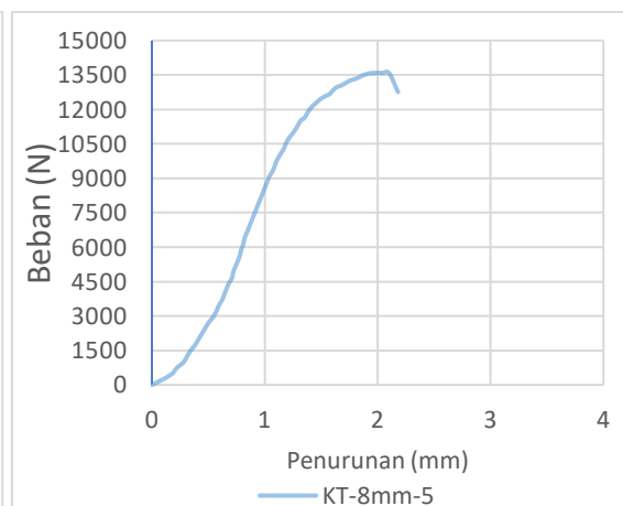
Grafik 7.6 Pengujian KT-8mm-5
