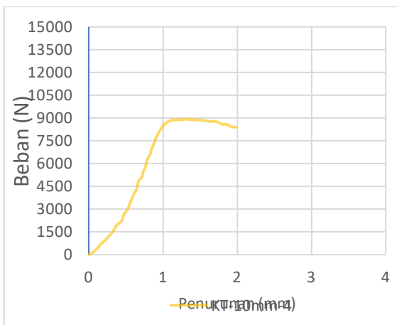
Grafik 7.11 Pengujian KT-10mm-4
