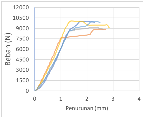
Grafik 7.13 Pengujiuan Kuat Tumpu dengan Baut Penekan 12mm
