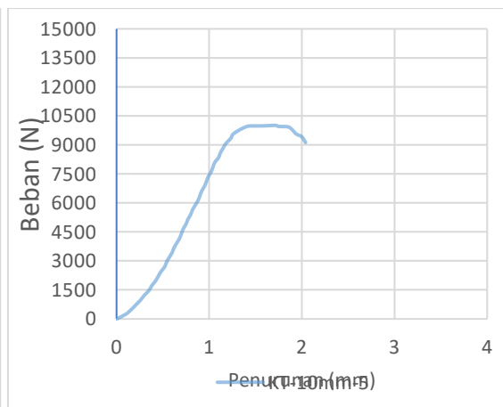
Grafik 7.12 Pengujian KT-10mm-5
