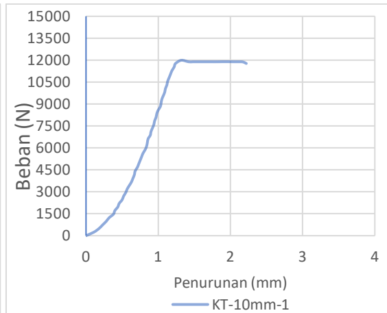
Grafik 7.8 Pengujian KT-10mm-1
