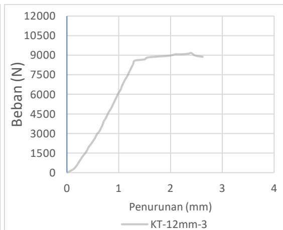
Grafik 7.16 Pengujiuan KT-12mm-3
