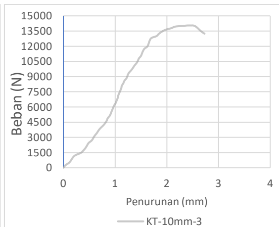
Grafik 7.10 Pengujian KT-10mm-3
