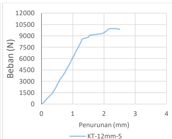
Grafik 7.18 Pengujiuan KT-12mm-5
