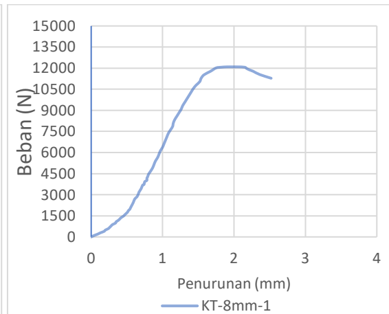
Grafik 7.2 Pengujian KT-8mm-1
