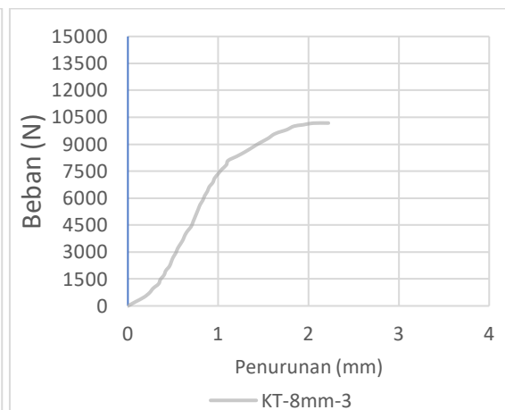
Grafik 7.4 Pengujian KT-8mm-3
