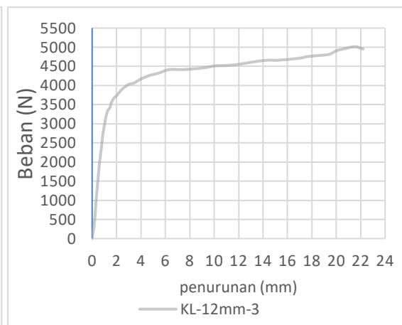
Grafik 6.16 Pengujian KL-12mm-3
