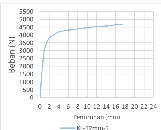
Grafik 6.18 Pengujian KL-12mm-5
