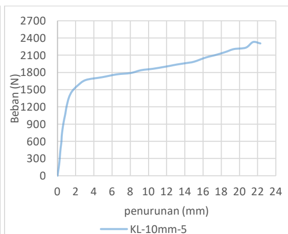
Grafik 6.12 Pengujian KL-10mm-5
