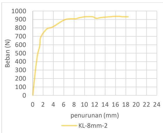
Grafik 6.3 Pengujian KL-8mm-2
