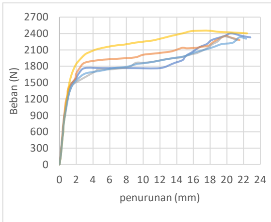
Grafik 6.7 Uji Kuat Lentur 10mm
