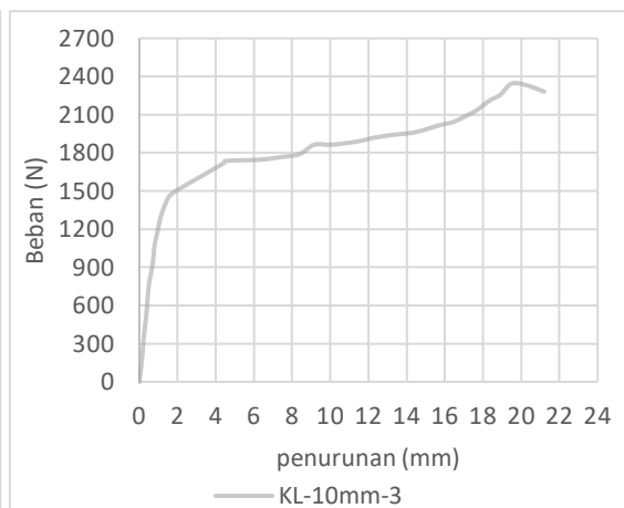
Grafik 6.10 Pengujian KL-10mm-3
