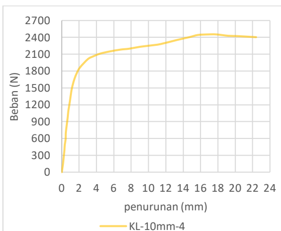
Grafik 6.11 Pengujian KL-10mm-4
