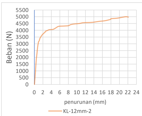
Grafik 6.15 Pengujian KL-12mm-2
