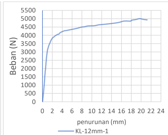
Grafik 6.14 Pengujian KL-12mm-1
