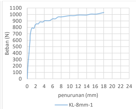
Grafik 6.2 Pengujian KL-8mm-1
