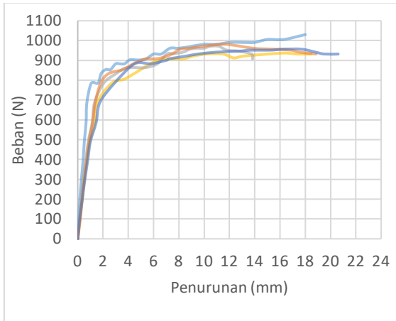
Grafik 6.1 Hasil Uji Kuat Lentur 8mm
