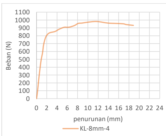
Grafik 6.5 Pengujian KL-8mm-4
