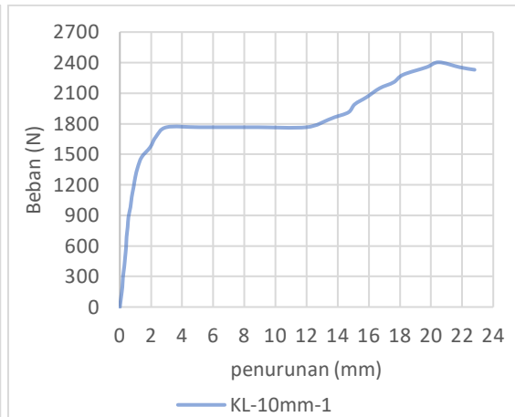
Grafik 6.8 Pengujian KL-10mm-1
