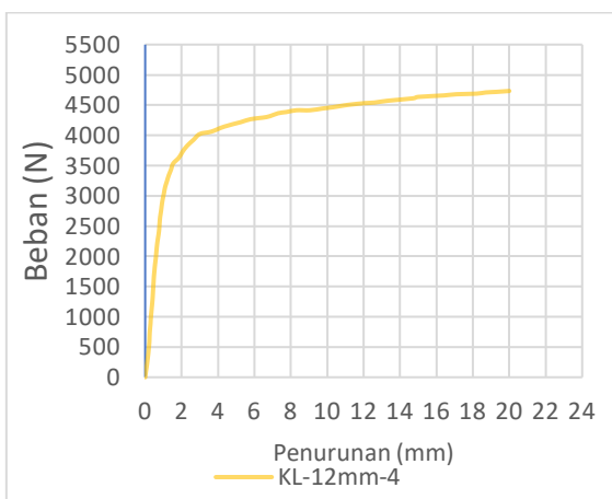
Grafik 6.17 Pengujian KL-12mm-4
