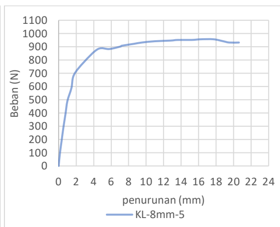
Grafik 6.6 Pengujian KL-8mm-5
