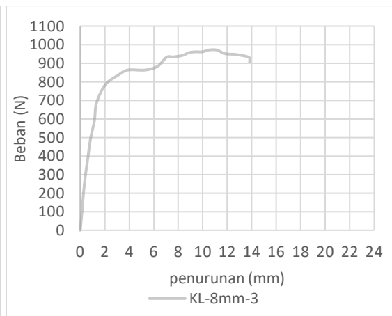
Grafik 6.4 Pengujian KL-8mm-3
