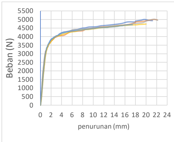
Grafik 6.13 Uji Kuat Lentur 12mm
