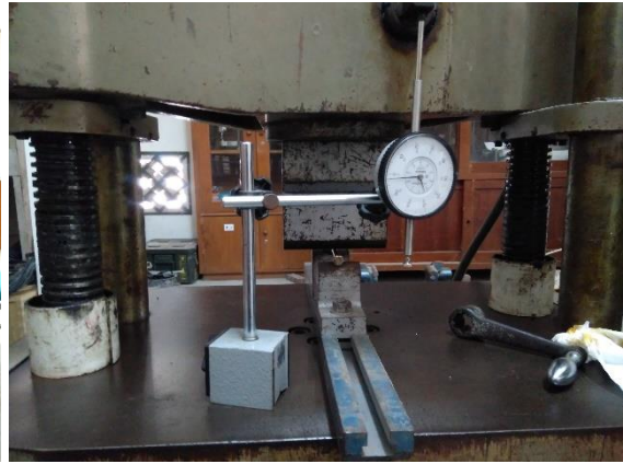
Gambar L-2.2. Uji KL-8mm-1
