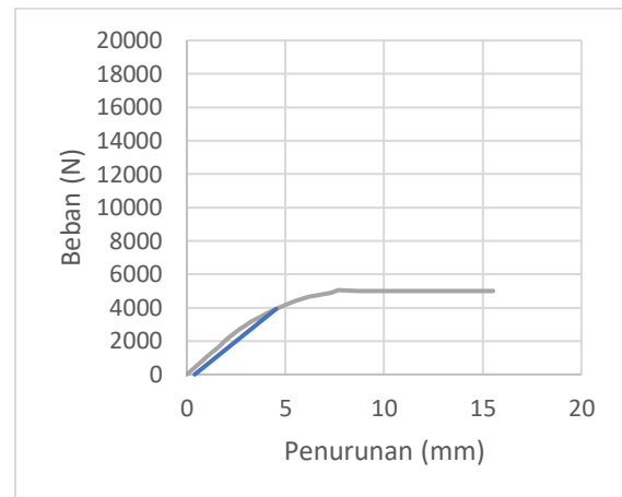
Grafik 14.4 KS-8mm-3 Terkoreksi
