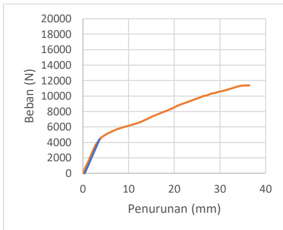
Grafik 14.3 KS-8mm-2 Terkoreksi
