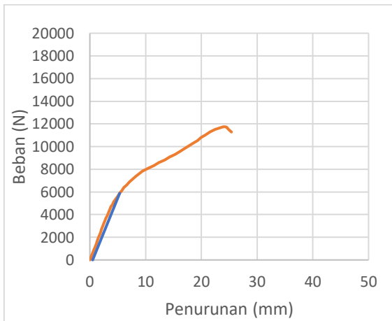
Grafik 14.9 KS-10mm-2 Terkoreksi
