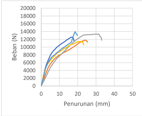
Grafik 14.7 Hasil Pengujian Kuat Sambung dengan Baut 10mm Terkoreksi
