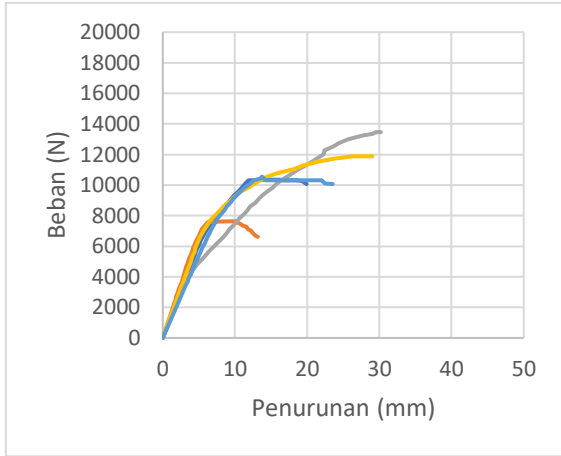
Grafik 14.13 Hasil Pengujian Kuat Sambung dengan Baut 12mm Terkoreksi
