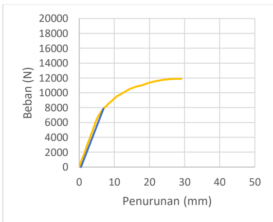
Grafik 14.17 KS-12mm-4 Terkoreksi
