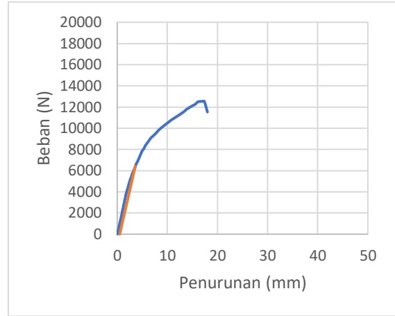
Grafik 14.8 KS-10mm-1 Terkoreksi
