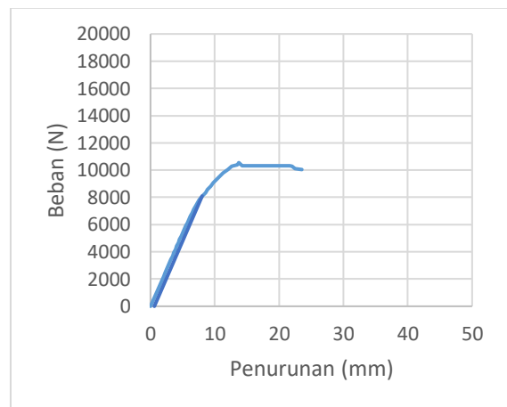
Grafik 14.18 KS-12mm-5 Terkoreksi
