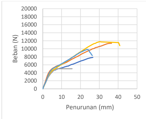
Grafik 14.1 Hasil Pengujian Kuat Sambung dengan Baut 8mm Terkoreksi
