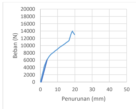
Grafik 14.12 KS-10mm-5 Terkoreksi
