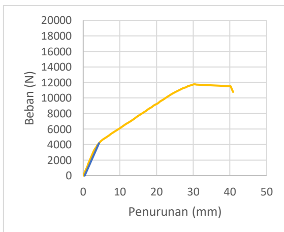
Grafik 14.5 KS-8mm-4 Terkoreksi
