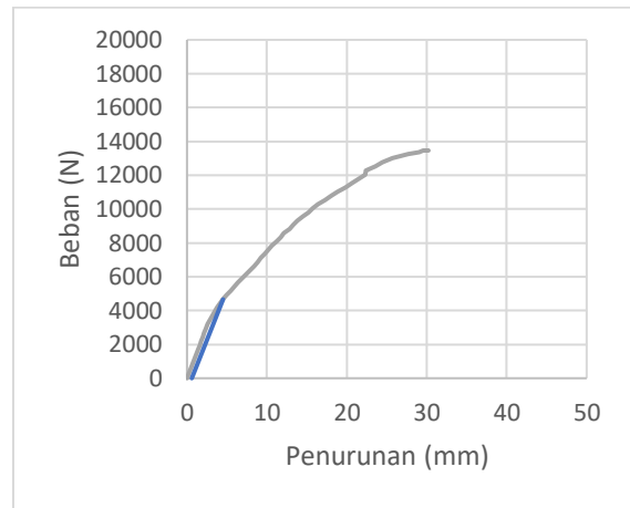
Grafik 14.16 KS-12mm-3 Terkoreksi
