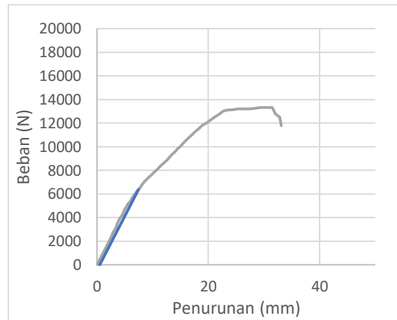
Grafik 14.10 KS-10mm-3 Terkoreksi
