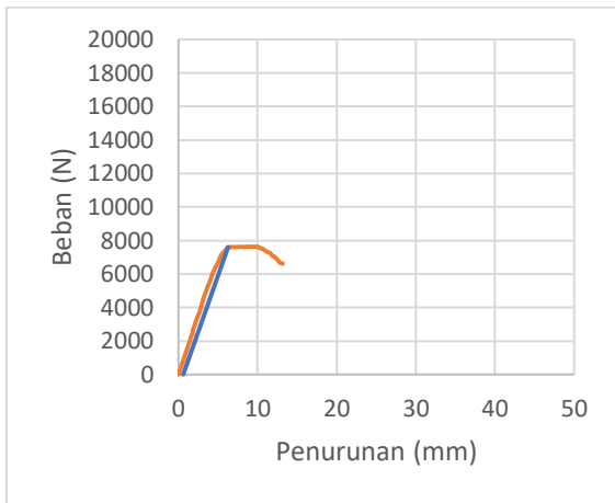
Grafik 14.15 KS-12mm-2 Terkoreksi
