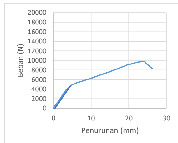
Grafik 14.6 KS-8mm-5 Terkoreksi
