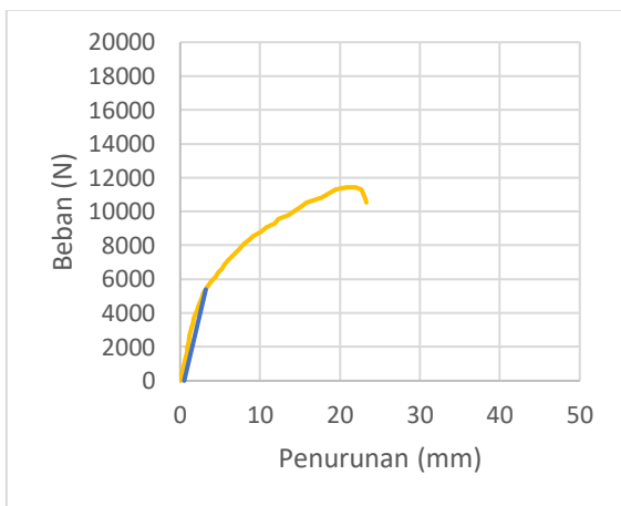
Grafik 14.11 KS-10mm-4 Terkoreksi
