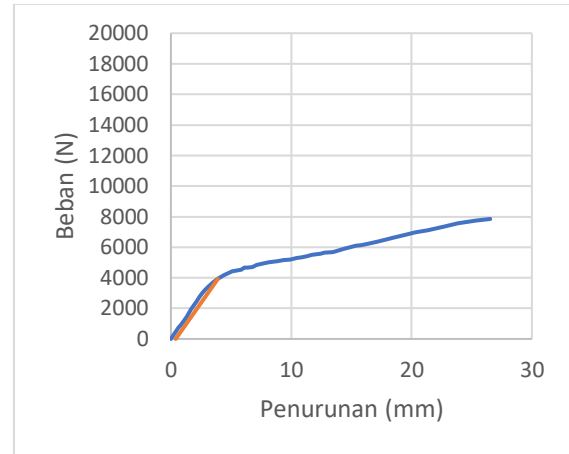
Grafik 14.2 KS-8mm-1 Terkoreksi
