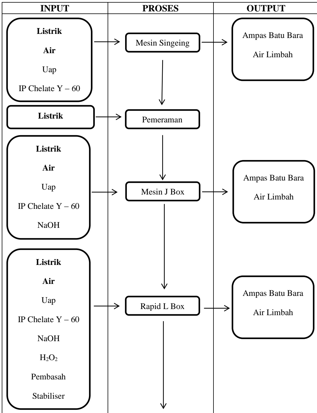
LAMPIRAN 2 - Alur Proses Produksi di Unit Finishing (1)
