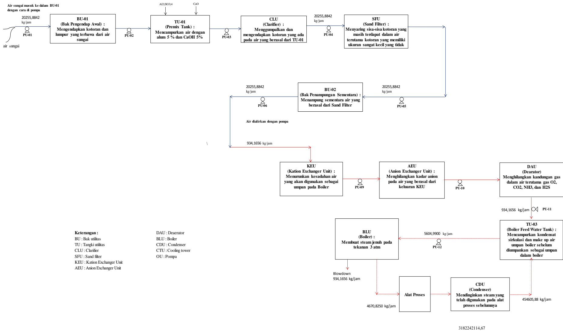
Gambar 4.7 Diagram Alir Pengolahan Air untuk Steam
