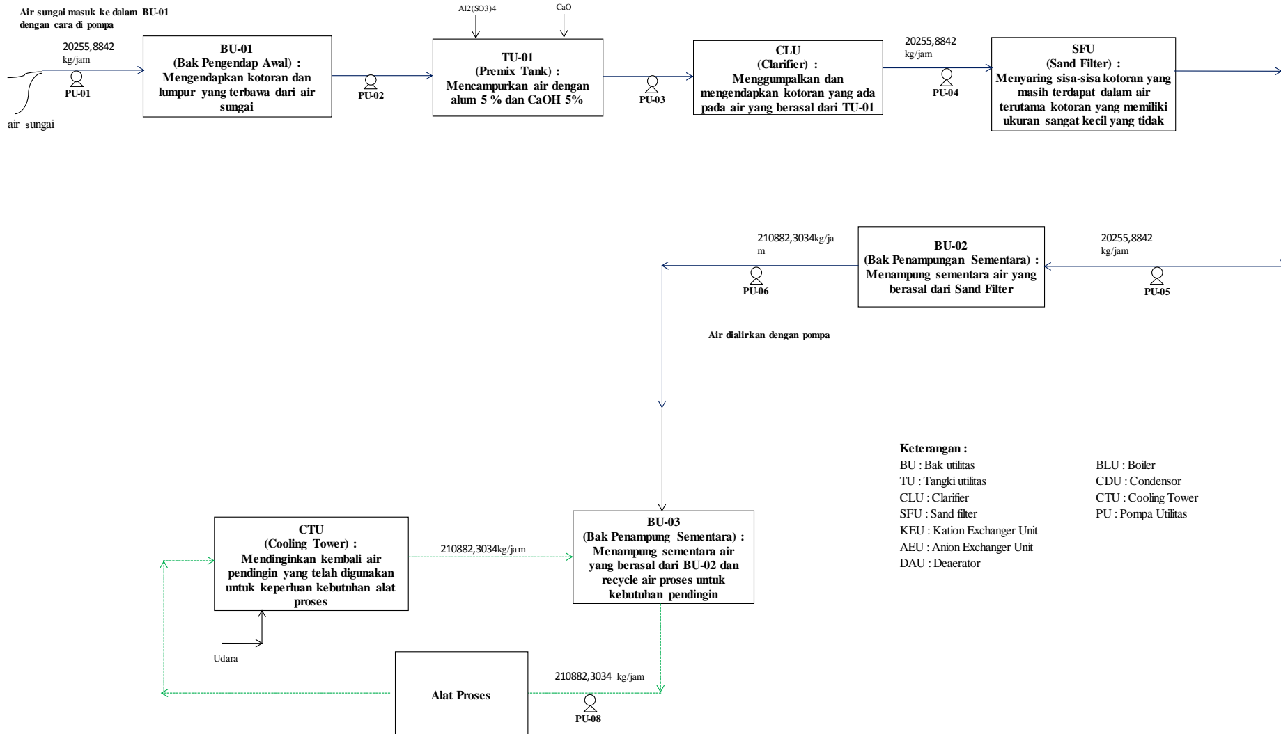
Gambar 4.8 Diagram Alir Pengolahan Air Untuk Pendingin
