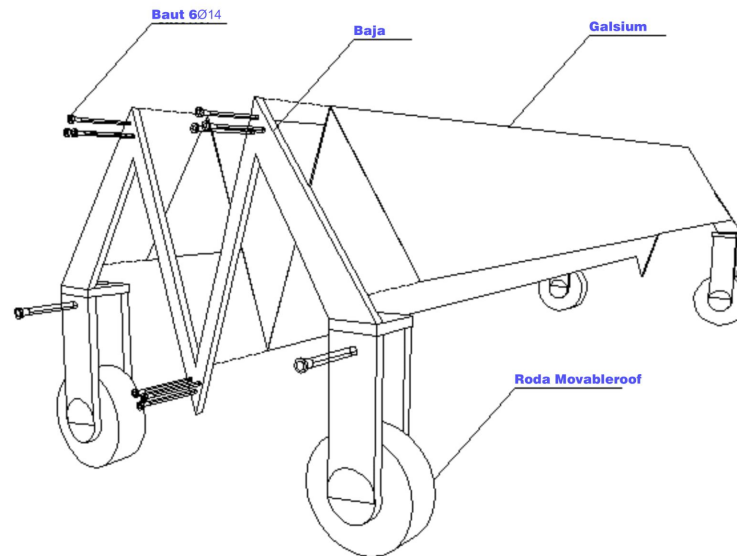
AKSONOMETRI DAN SAMBUNGAN
