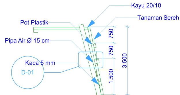
Potongan A-A' Skala 1 : 50
