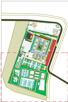
Masterplane Skala 1 : 2000
