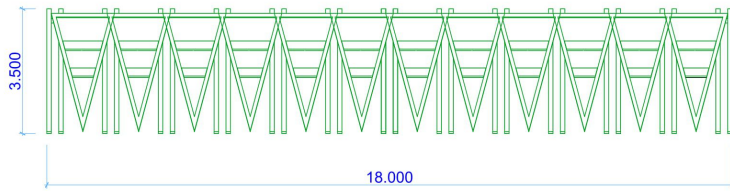
Tampak Samping Skala 1 : 100
