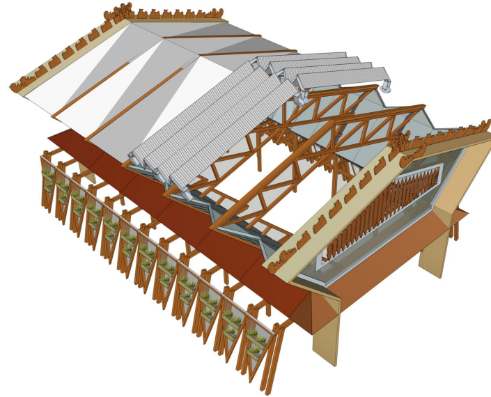
Movableroof Posisi Terbuka
