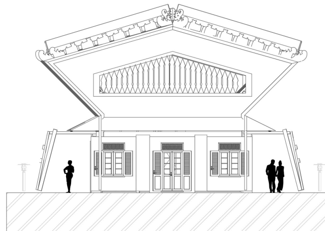
Tampak Selatan Skala 1 : 100
