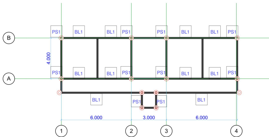
SRUKTUR PONDASI BUNGALOW RESORT Skala 1 : 100
