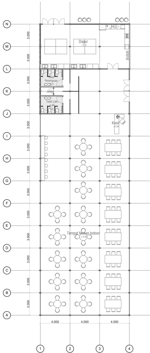
RESTORAN IKAN AIR TAWAR Skala 1 : 150
