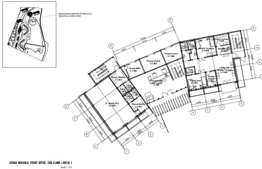
Gambar 7 . 3 Redesain Denah Mushola, Klinik, dan Front Office
