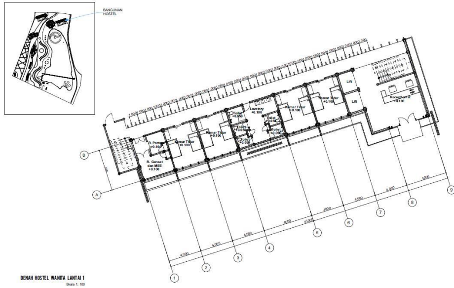
Gambar 7. 1 Redesain Denah Hostel Wanita dan Pria
