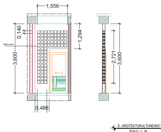
Gambar 6.1: Detail Dinding Sumber: Penulis, 2018
