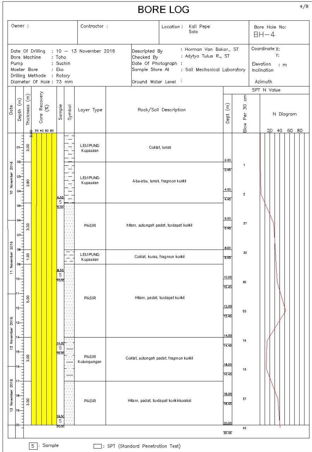
Gambar L-1.1 Grafik SPT BH-4
