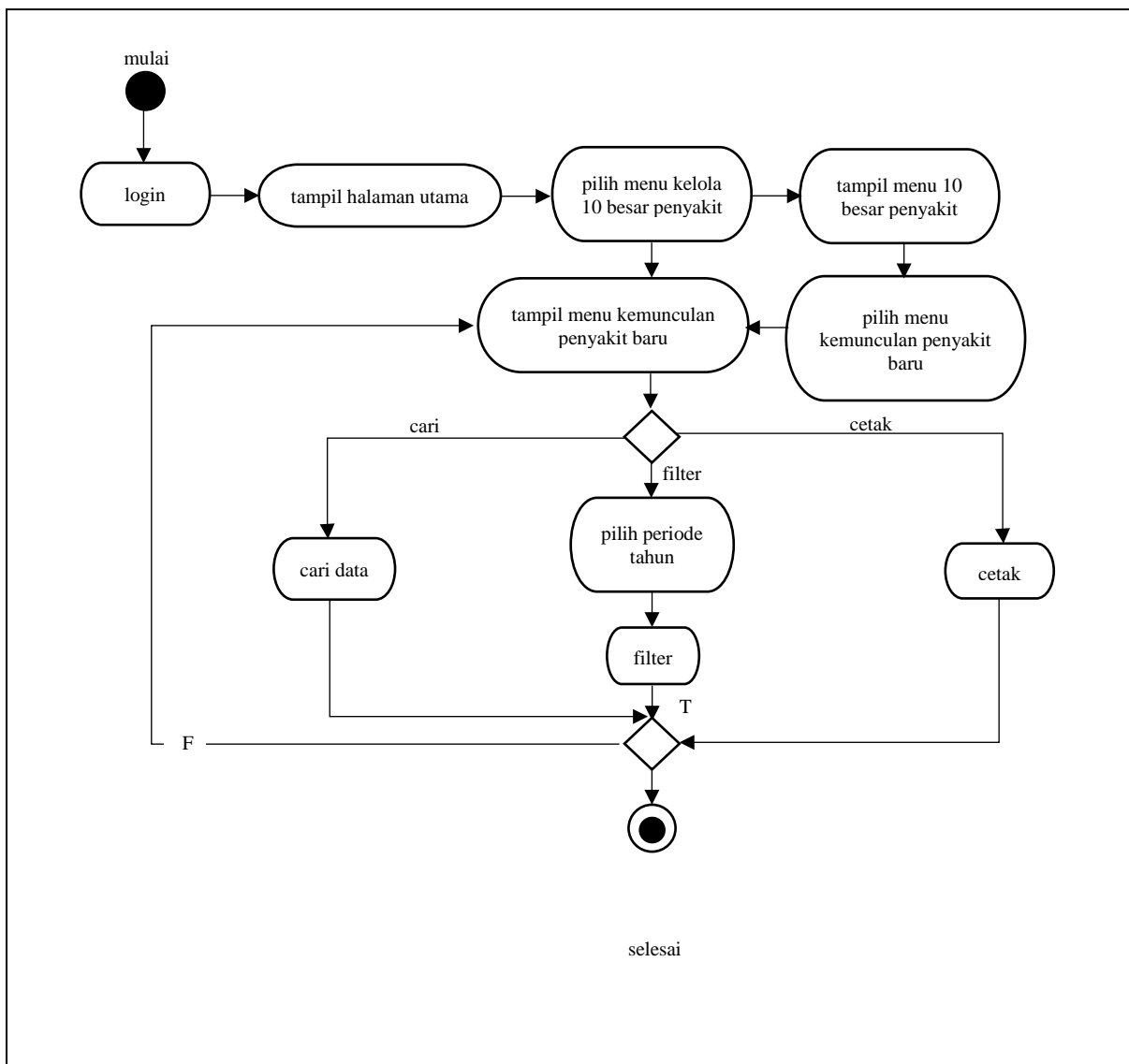
Gambar 3.16 Activity Diagram Kemunculan Penyakit Baru
