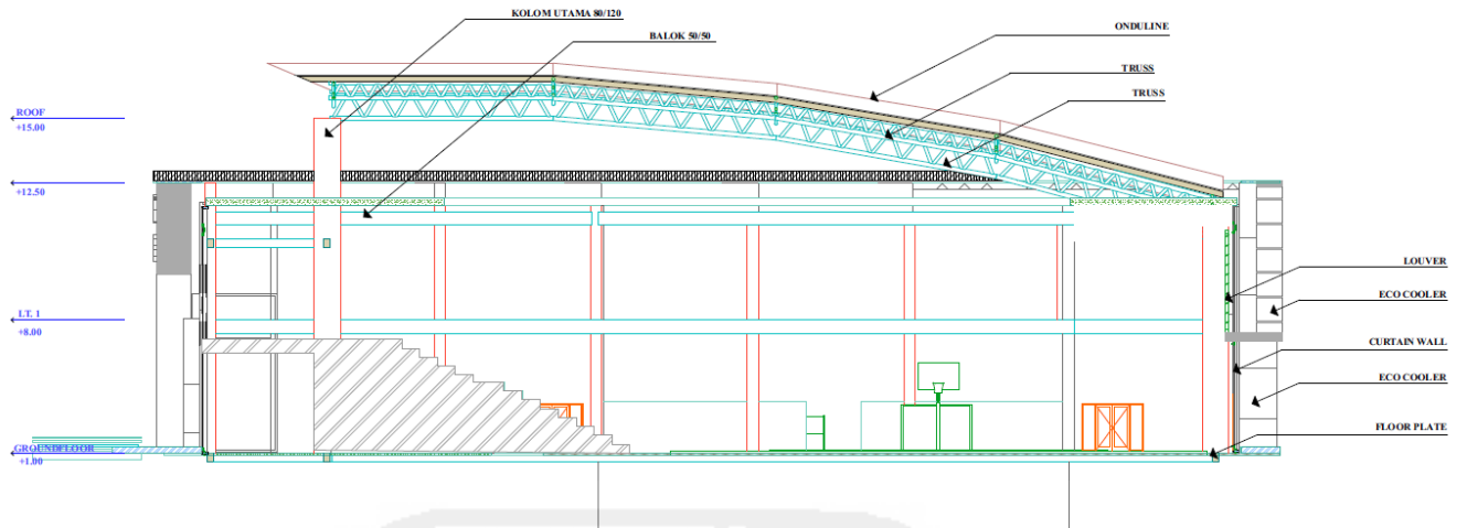
Gambar 4. 4 potongan B-B
