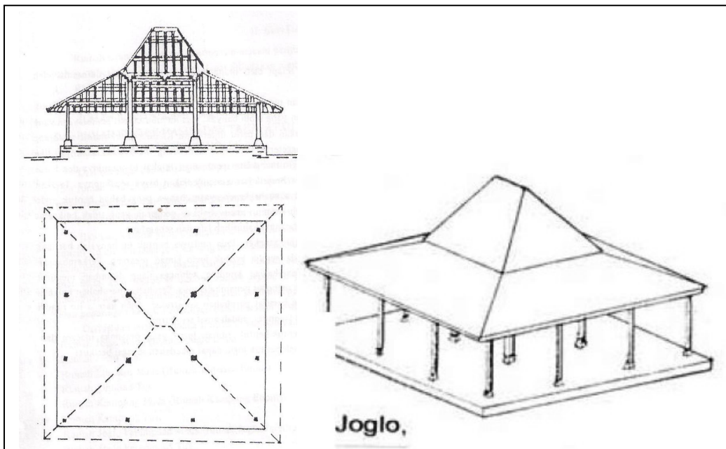
Gambar 23. Rumah Joglo Sumber : Drs.Hamzuri
