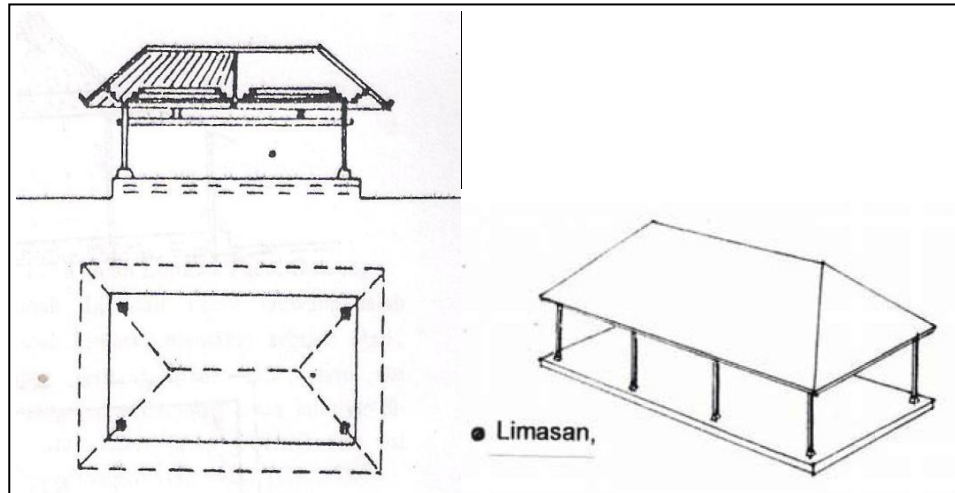
Gambar 22. Rumah bentuk Limasan Sumber : Drs. Hamzuri
