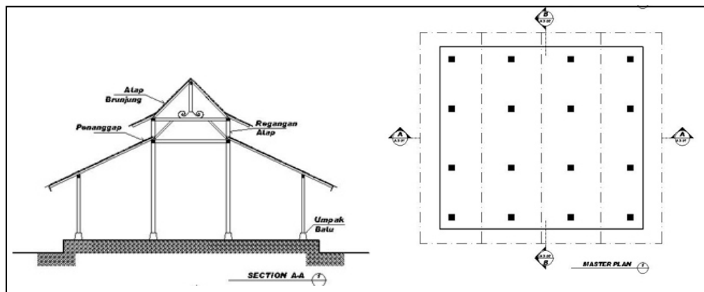
Gambar 21. Rumah Kampung Lambang Teplok Sumber : Google Image
