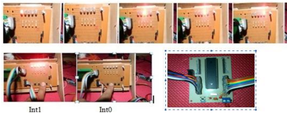
Gambar 4. 13 Interupsi Eksternal
