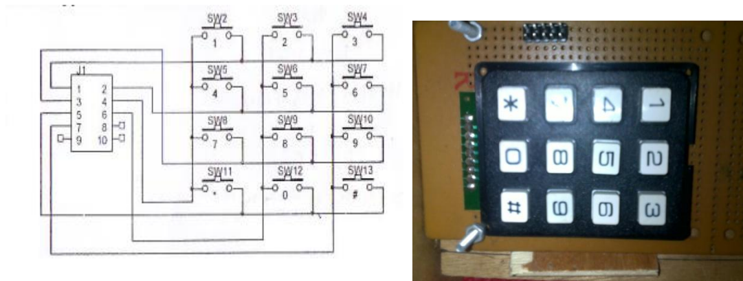
Gambar 3. 9 Rangkaian Keypad
