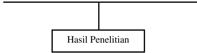
Gambar 2.1 Kerangka Pikir
