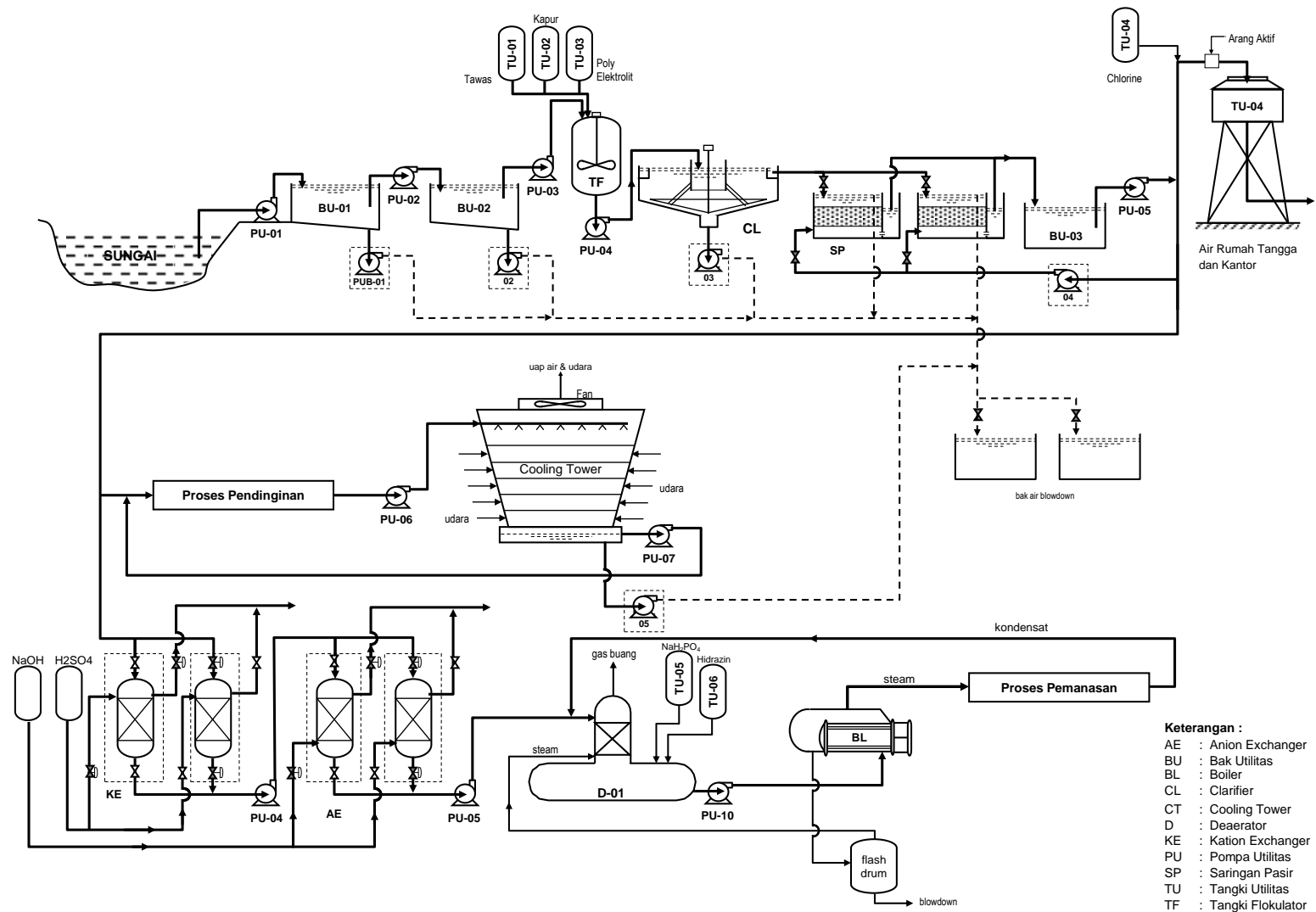
Gambar Skema Unit Pengolahan Air
