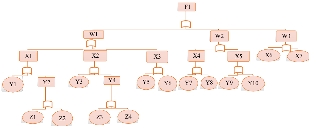
Gambar 5 FTA ( Fault Tree Analysis ) Resiko Pekerja Sesak Nafas pada pekerjaan Pembersihan Shat Lift pada Konstruksi Lift (F1)
