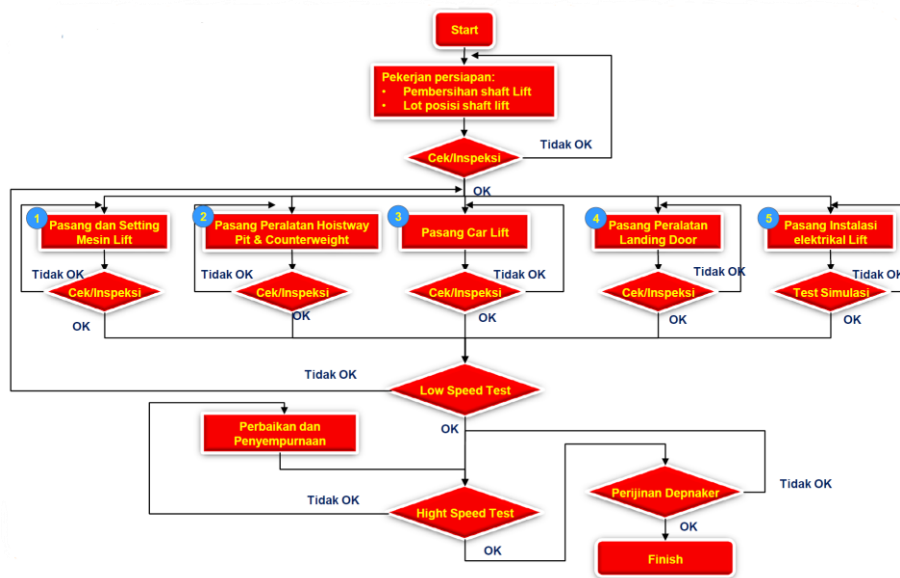
Gambar 3 Metode Pelaksanaan Konstruksi Lift
