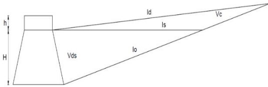
Gambar 1. Sketsa kapasitas tampungan sabo dam
