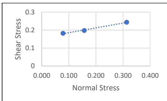
Gambar 5. Grafik kuat geser langsung
