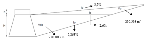
Gambar 6. Sketsa hasil analisis kapasitas tampungan sabo dam GE-C13
