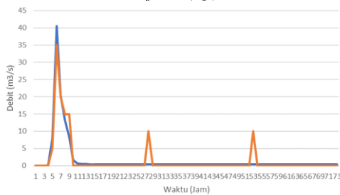
Gambar 14 Pola Operasi Pompa ( Q_2 )
