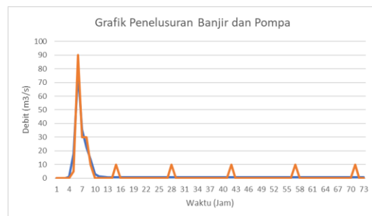
Gambar 18 Pola Operasi Pompa ( Q_{25} )
