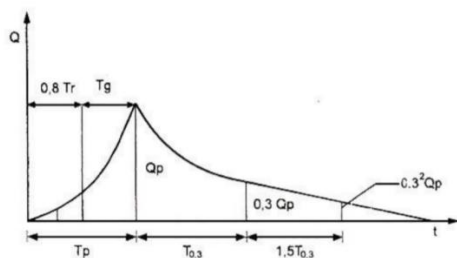
Gambar 2 Hidrograf Satuan Sintetis Nakayasu
