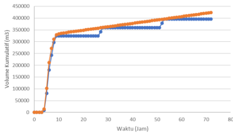
Gambar 13 Grafik Hubungan antara inflow dan outflow ( Q_2 )
