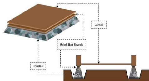
Gambar 4. Kaki Rumah
