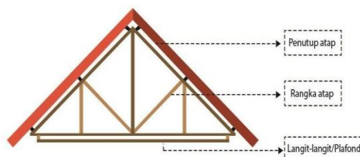
Gambar 2. Penutup Atap
