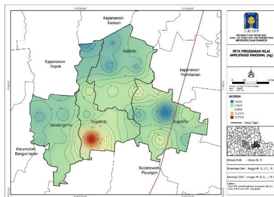
Gambar 9. Peta Persebaran Faktor Amplifikasi Tanah (Ag)
