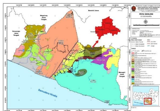
Gambar 1. Kondisi Geologi Kecamatan Berbah
