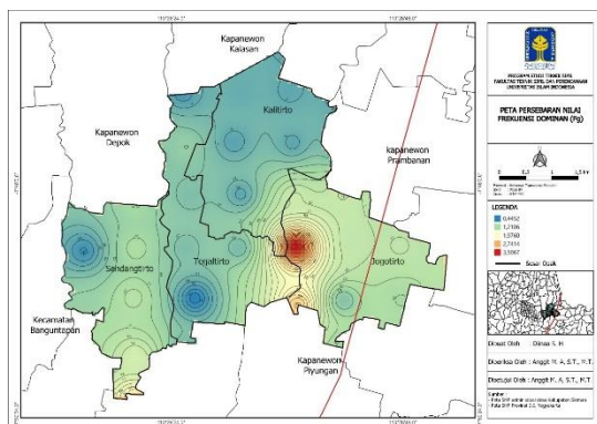
Gambar 10. Peta Persebaran Nilai Frekuensi Dominan Tanah (Fg)
