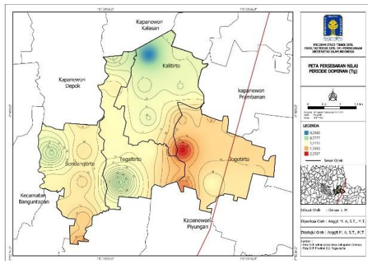
Gambar 11. Peta Persebaran Nilai Periode Dominan Tanah (Tg)
