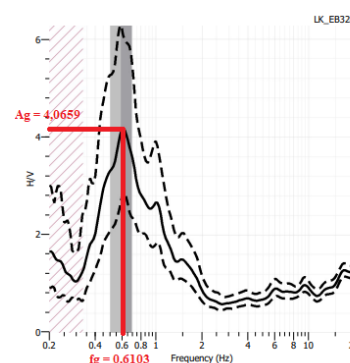
Gambar 8. Nilai Puncak Kurva HVSR Pada Titik 1
