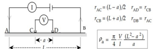
Gambar 3. Konfigurasi schlumberger
