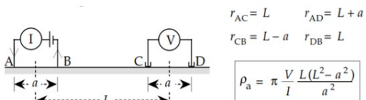
Gambar 4 Konfigurasi dipole-dipole
