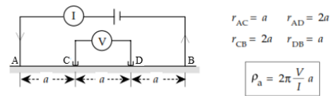
Gambar 2. Konfigurasi wenner
