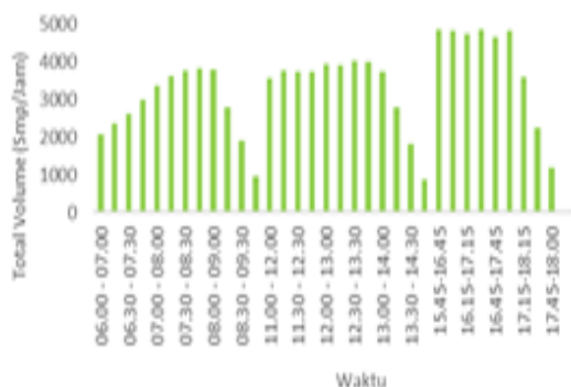
Gambar 3 Grafik Volume Lalu Lintas Simpang Monjali Hari Sabtu
