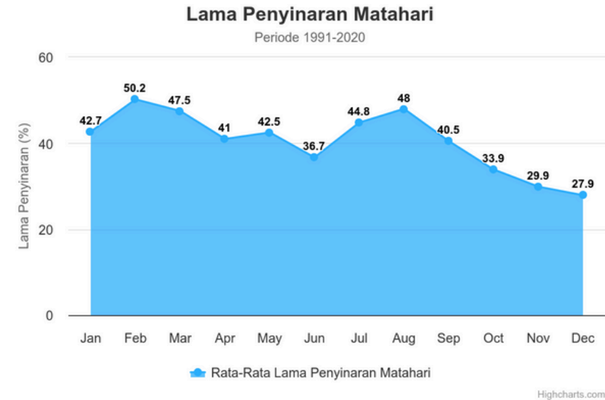
Gambar 19.0 Data rata-rata penyinaran matahari Sumber : https://www.meteoblue.com
