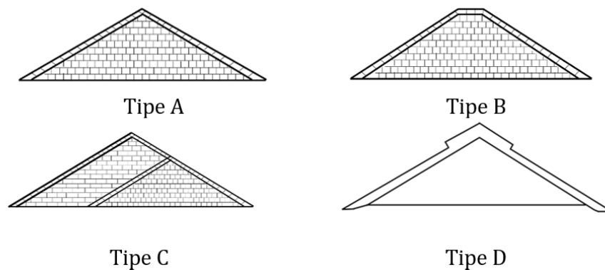
Gambar 2 Tipe atap bangunan Indish
