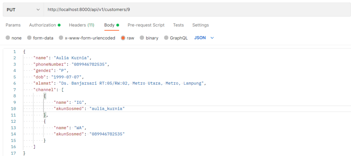
Gambar 3.20 Body Request Untuk Mengubah Data Customer
