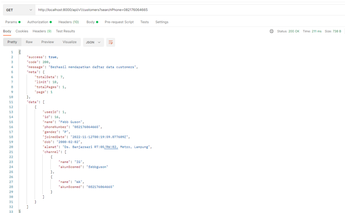
Gambar 3.24 Response Mencari Data Customer Berdasarkan Nomor Telepon
