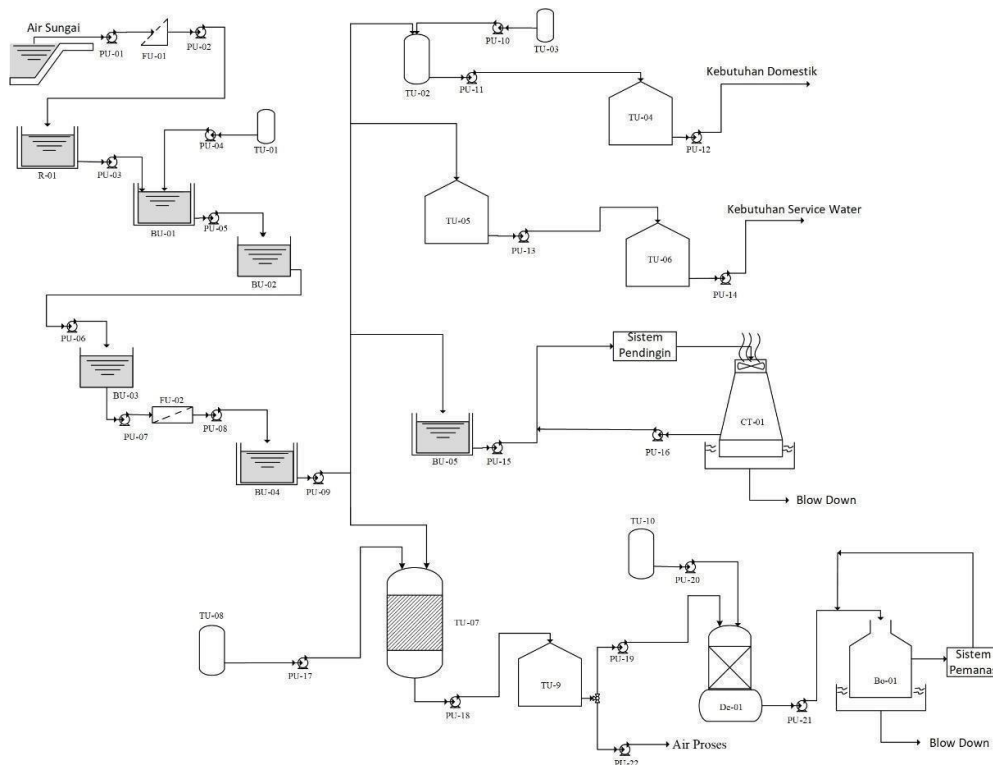
Gambar 4.7 Unit Utilitas
