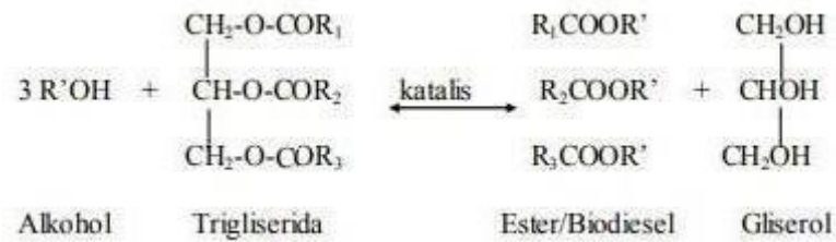
Gambar 3.2 Reaksi Transesterifikasi
