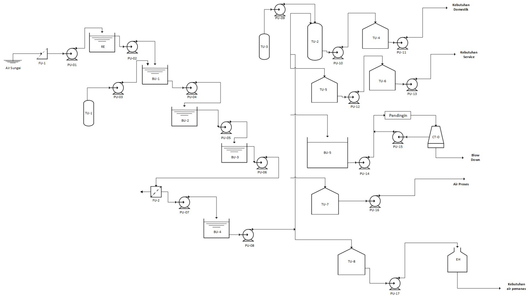
Gambar 5.1 Unit Utilitas
