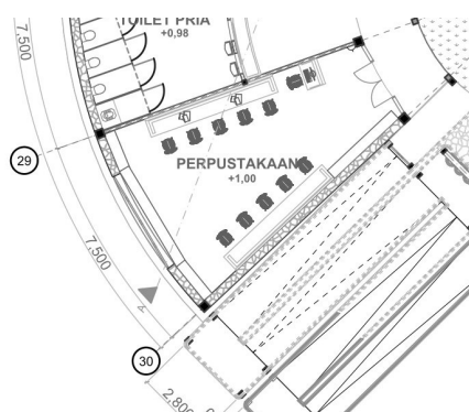
Gambar 4.85 Detail Denah Perpustakaan Sumber : Penulis, 2023
