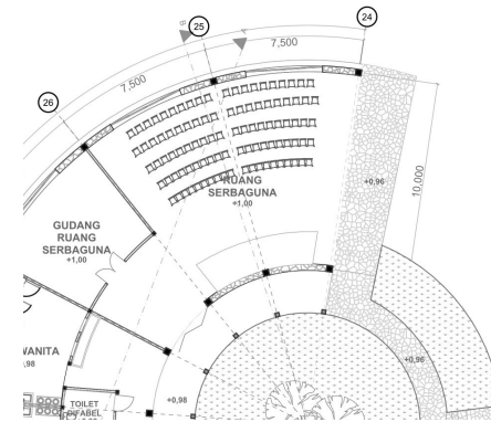
Gambar 4.88 Detail Denah Ruang Serbaguna Sumber : Penulis, 2023
