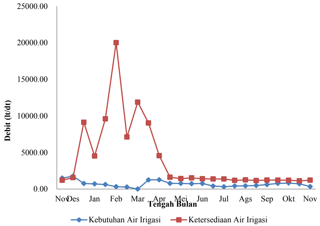
Gambar 5.14 Kesesimbangan Air Alternatif 4 (Sumber : Analisis data, 2015)
