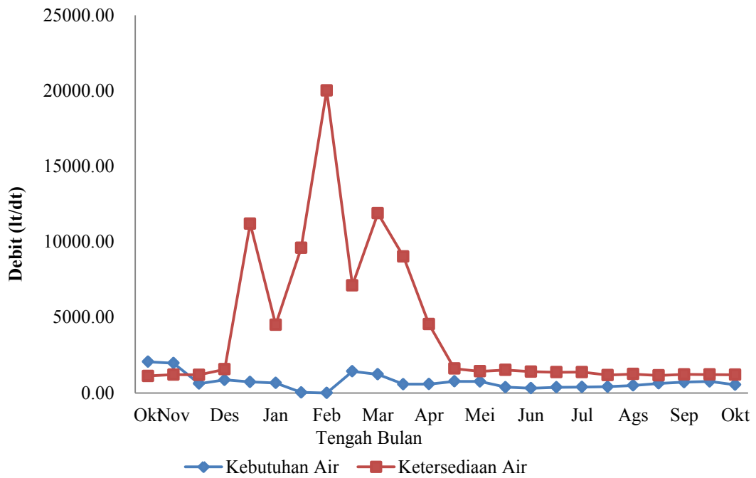
Gambar 5.12 Kestimbangan Air Alternatif 2 (Sumber : Analisis data, 2015)
