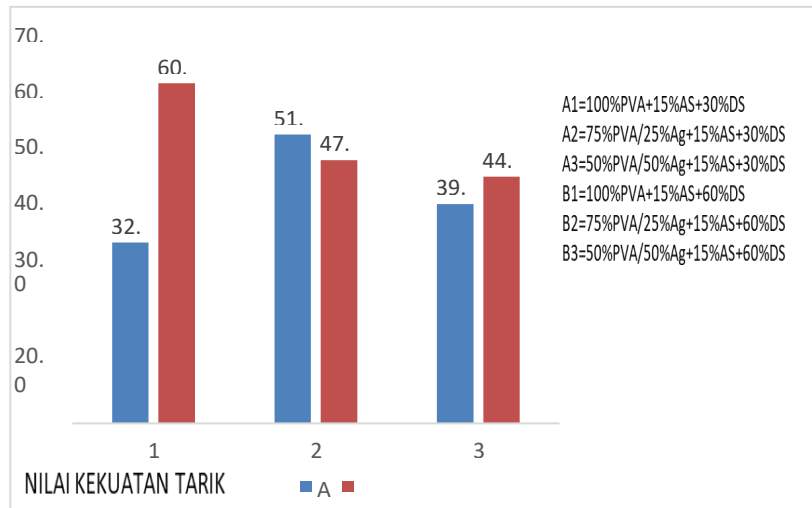
Gambar 4. 2 Nilai uji kekuatan tarik.
