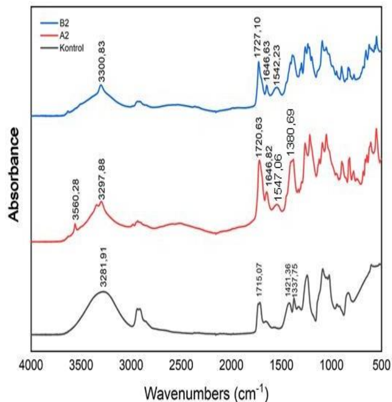
Gambar 4. 5 Grafik FTIR
