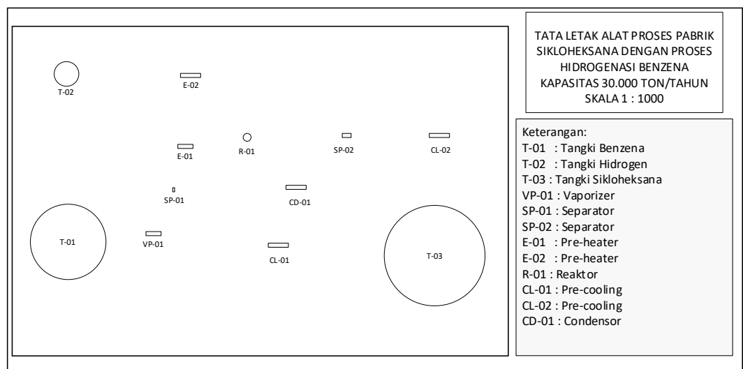
Gambar 4.3 Tata Letak Alat Proses
