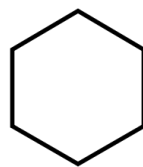
Gambar 1.10 Struktur kimia Sikloheksana
