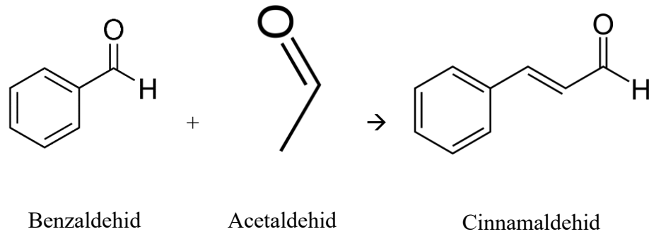
Gambar 1. 4 Reaksi Pembentukan Cinnamaldehyd
