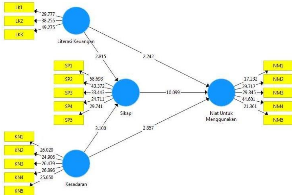
Gambar 4.3 Pengujian Hipotesis
