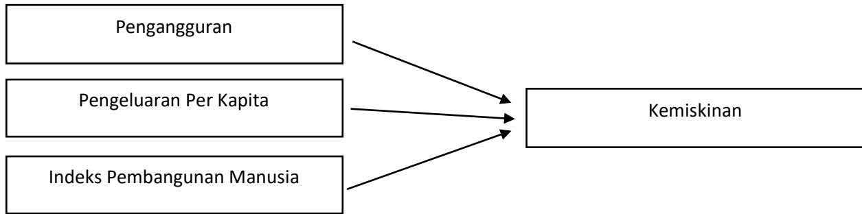
Gambar 2. 1 Kerangka Pemikiran
