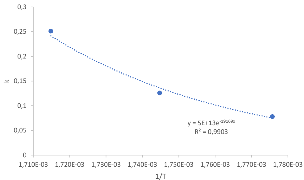
Gambar 1.5 Grafik Kinetika
