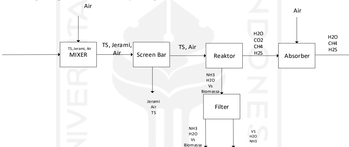
Gambar 3. 1 Diagram proses terbentuknya biogas
