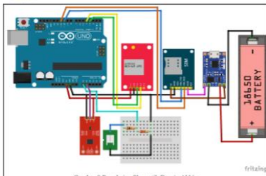
Gambar 9 Rangkaian Skematik Desain Akhir.
