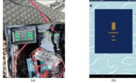
Gambar 3.2 Sisa baterai awal pada voltmeter (a) dan pada aplikasi EMOT (b) rate kutup. Hasil pengujian yang ditunjukkan dengan Gambar 3.2 terdapat perbedaan pembacaan antara voltmeter dengan aplikasi, oleh sebab itu didapatkan persentase kesalahan pembacaan sebagai berikut.
