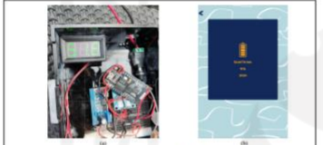
Gambar 2.2 Sisa baterai awal pada voltmeter (a) dan pada aplikasi EMOT (b) saat awal.
