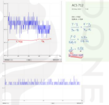
Menggabungkan sensor arus dan pembagi tegangan
