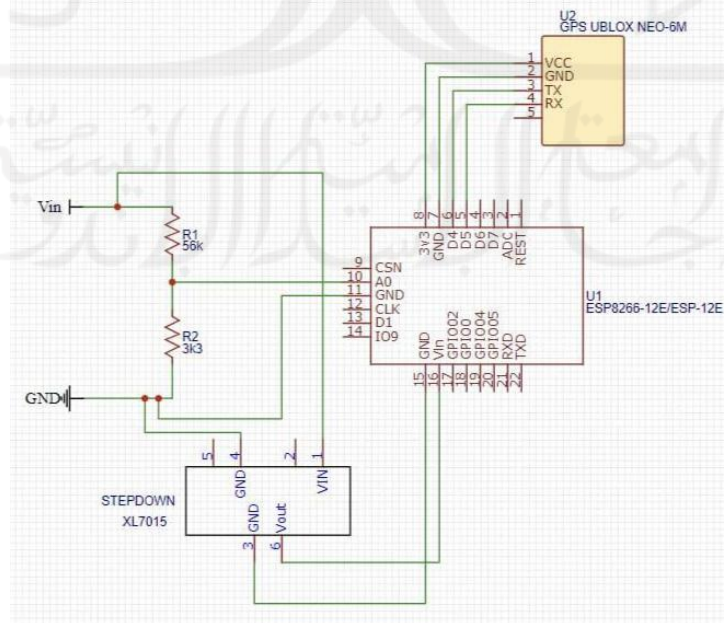
Gambar 3.6. Skematik rangkaian
