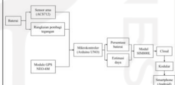
Gambar 8 Blok Diagram Desain Akhir.
