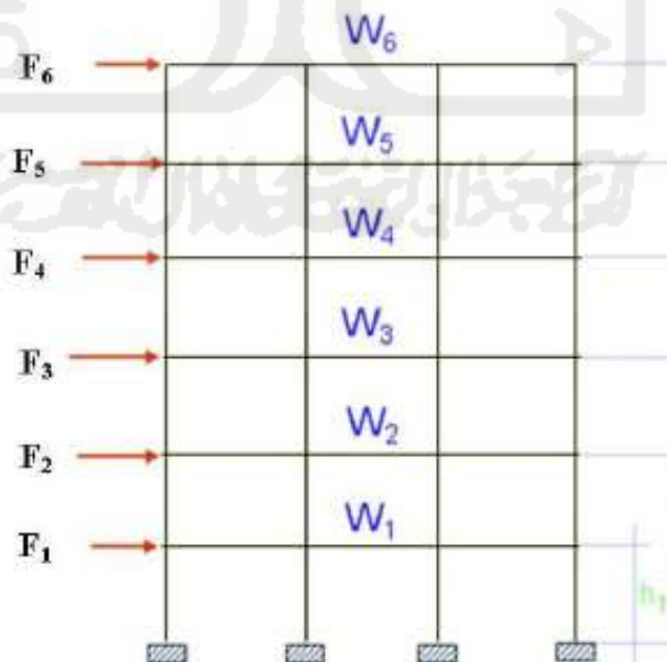
Gambar 3.5 Penempatan gaya lateral ekuivalen. (SNI 03-1726-2012)
