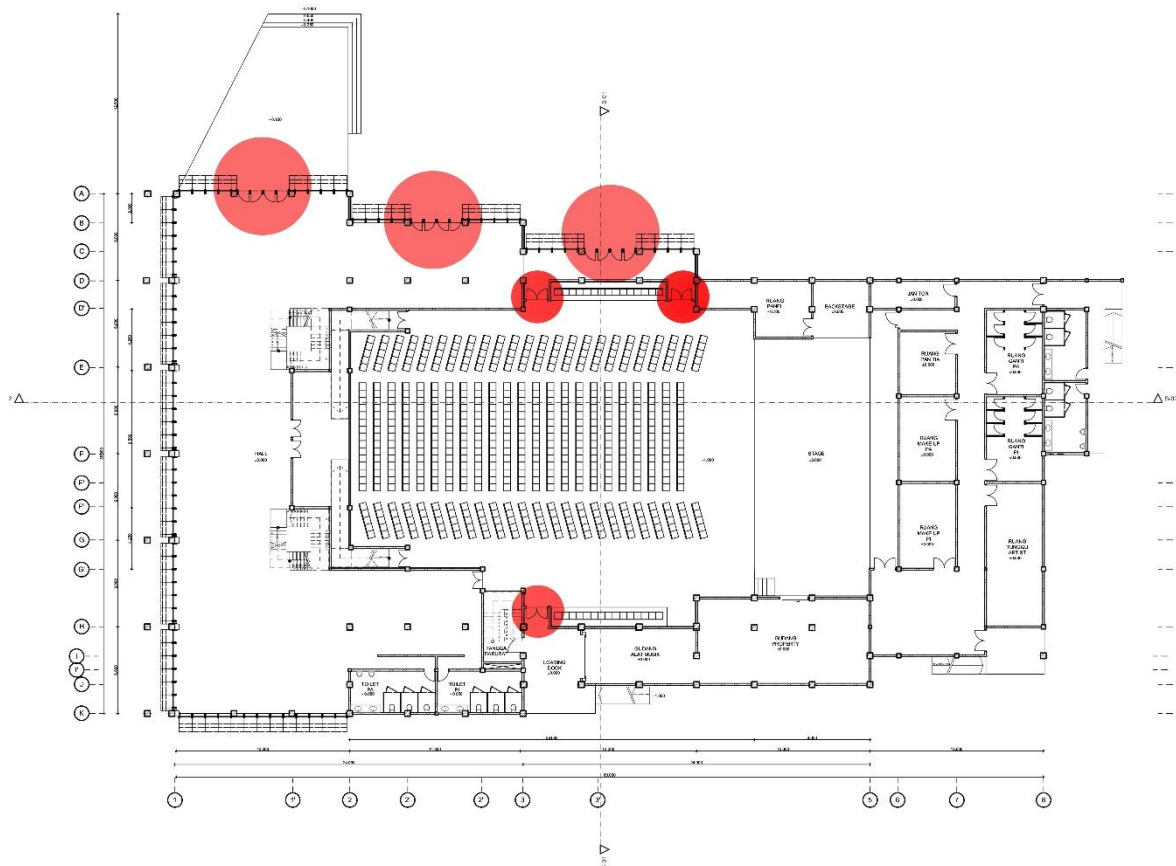
Gambar 5.2. Skema keselamatan tambahan pintu exit dalam bangunan dan luar
