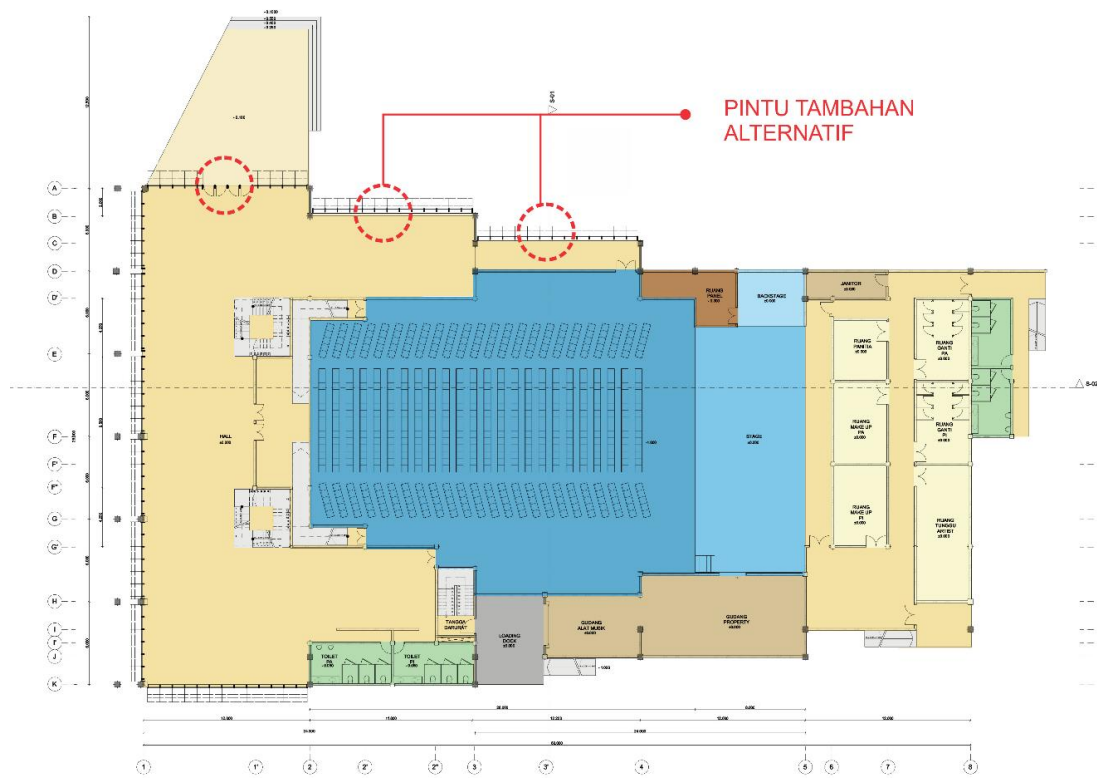
Gambar 5.1. Skema Keselamatan Tambahan Pintu Exit
