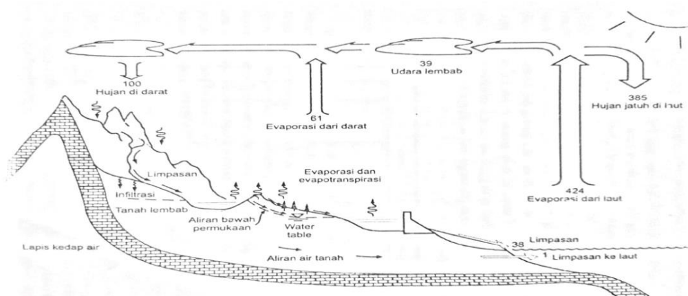
Gambar 3.1 Siklus Hidrologi
