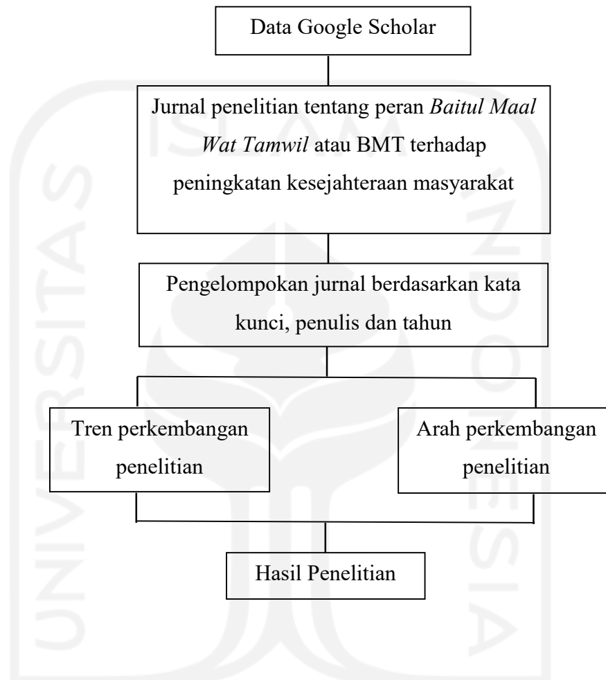
Gambar 1 Kerangka Berpikir
