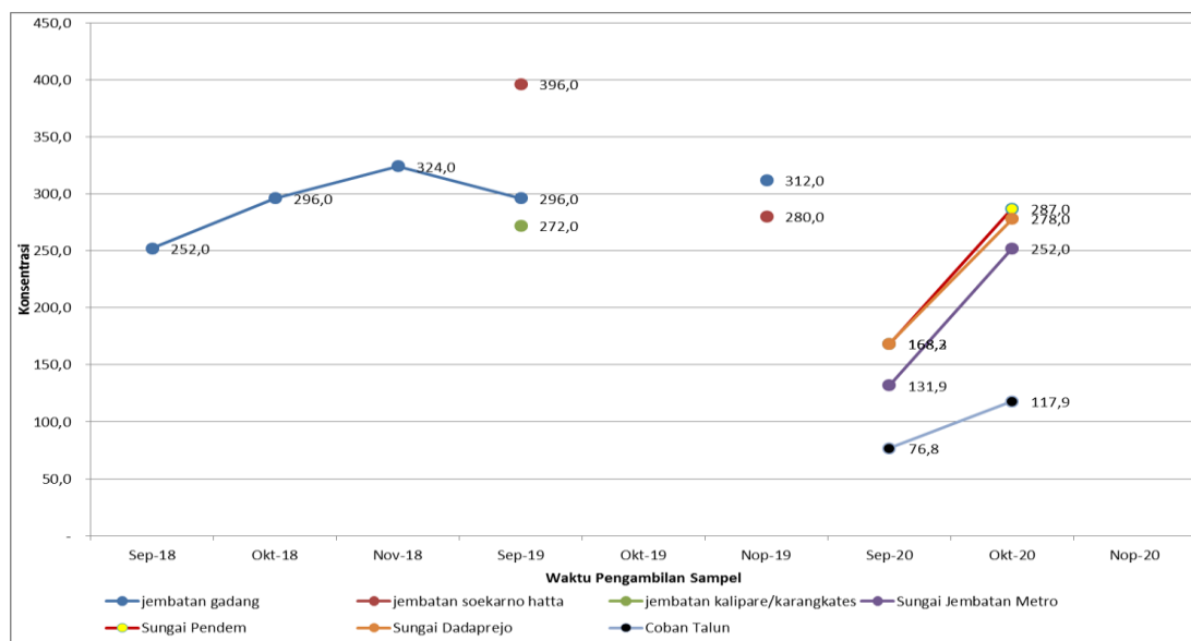
Gambar 7 Grafik Perubahan Konsentrasi TDS terhadap Waktu
