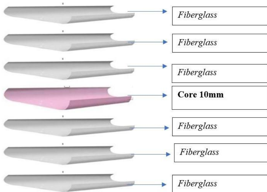
Gambar 3. 16 Komposisi Komposit Sandwich
