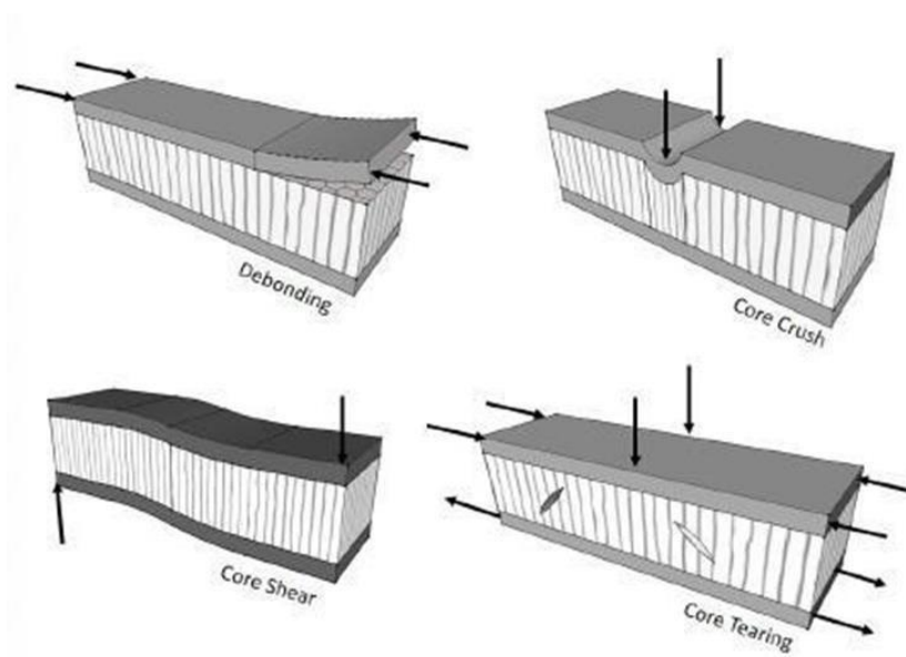
Gambar 2. 9 Jenis-jenis Kegagalan Pada Core Komposit Sandwich
