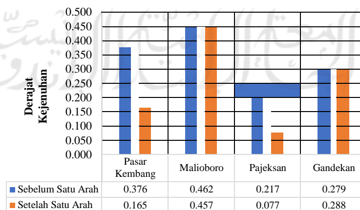
Gambar 5.34 Diagram Perbandingan Derajat Kejenuhan
